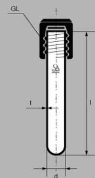
1231-S 罗口试管
