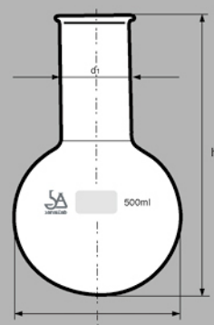
1115 圆底烧瓶 长颈
